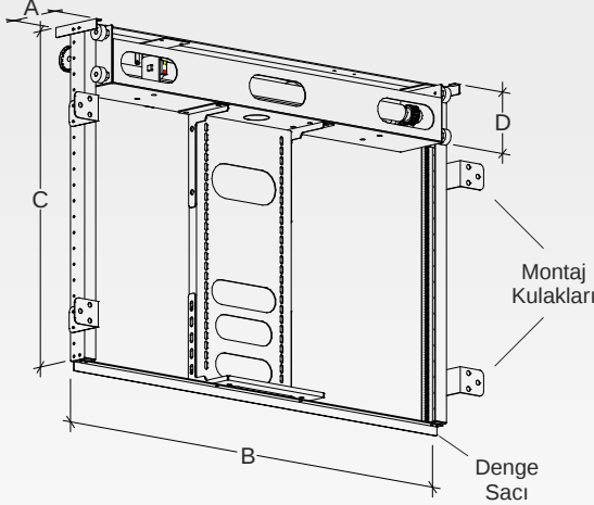
KAPALI GÖRÜNÜM
