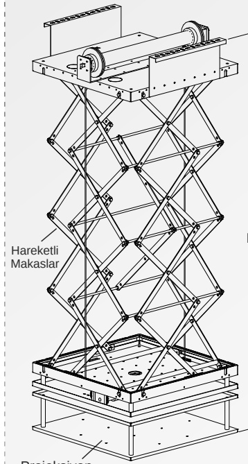
AÇIK GÖRÜNÜM
