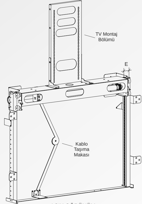
AÇIK GÖRÜNÜM
