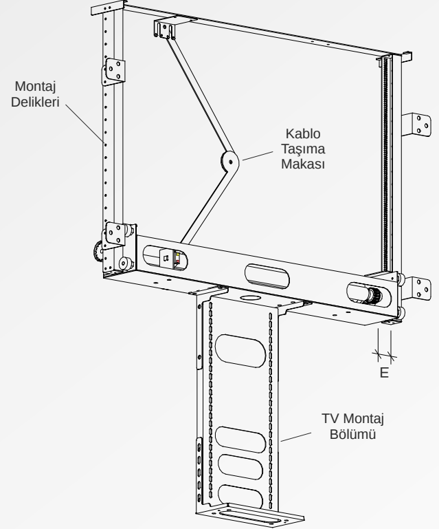
AÇIK GÖRÜNÜM
