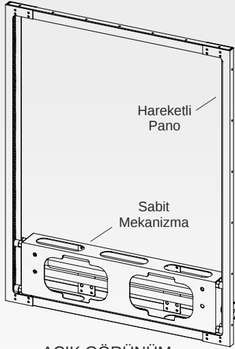
AÇIK GÖRÜNÜM
