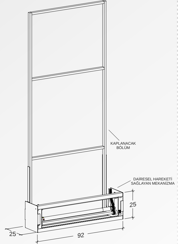
KAPALI GÖRÜNÜM
