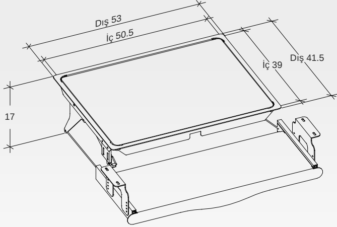
KAPALI GÖRÜNÜM
