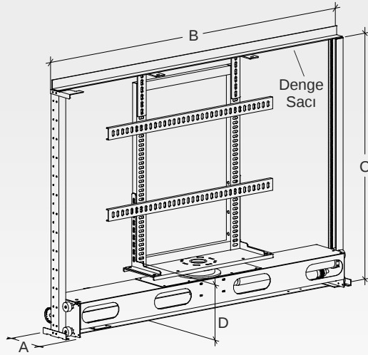
KAPALI GÖRÜNÜM
