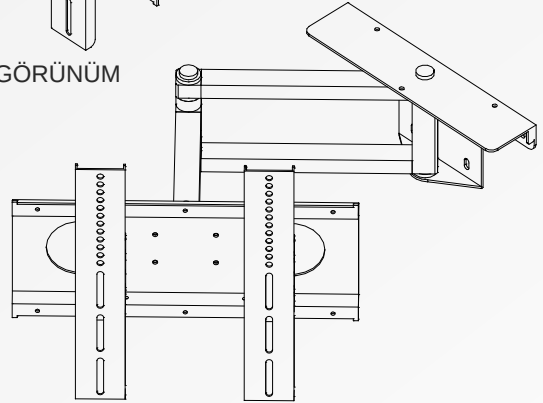
AÇIK GÖRÜNÜM
