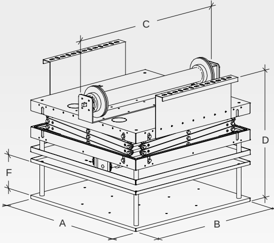
KAPALI GÖRÜNÜM
