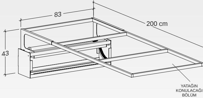
AÇIK GÖRÜNÜM
