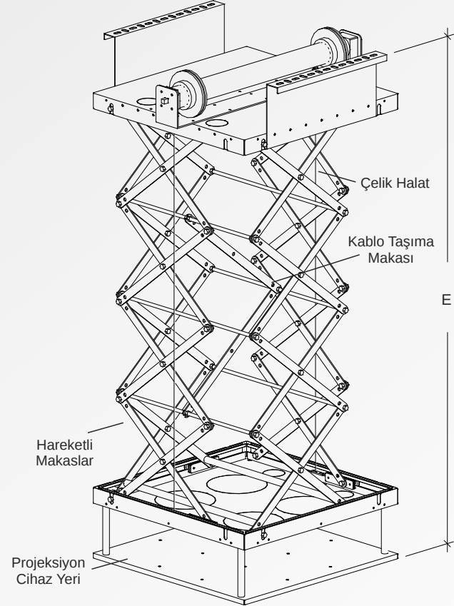
AÇIK GÖRÜNÜM
